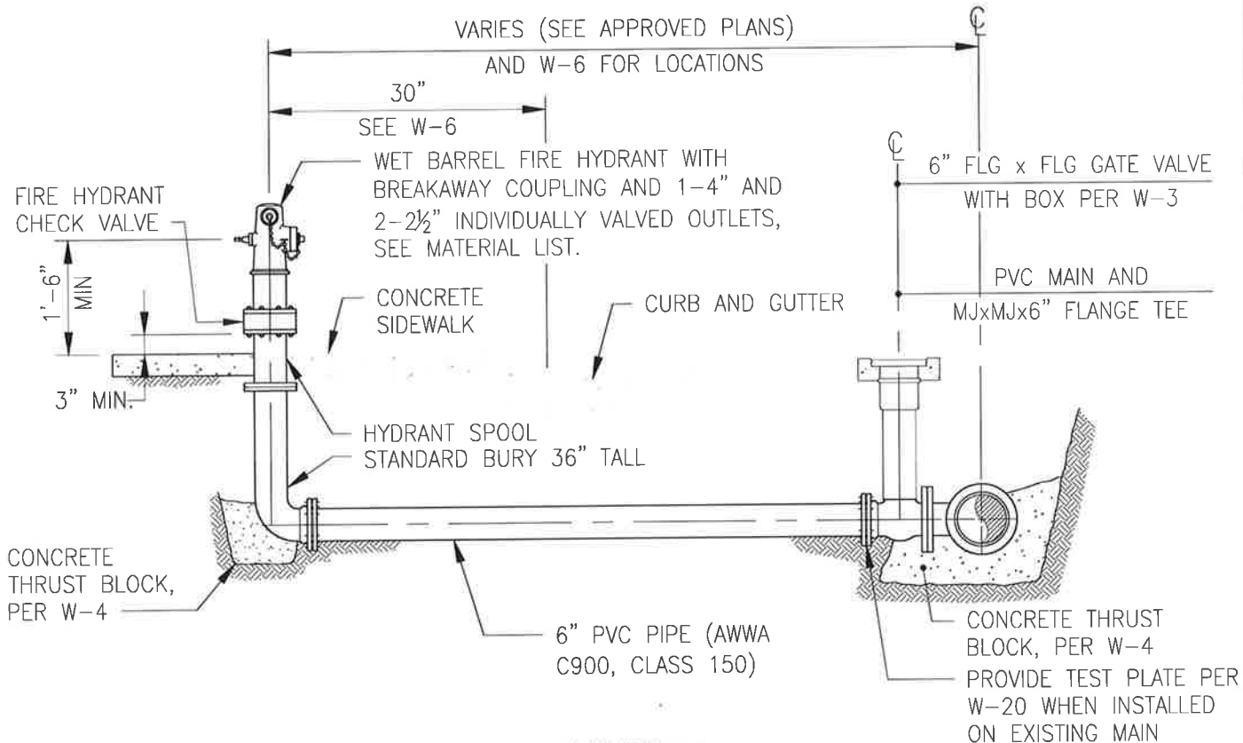
ELEVATION
