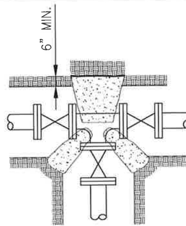
MAINLINE TEE
